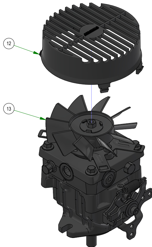
050-3001-00 & 050-3003-00 PUMP ASSEMBLIES
