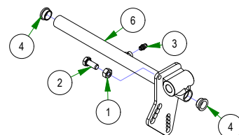
031-0054-21 2021 Maverick Drive Arm Actuator LH Assembly
