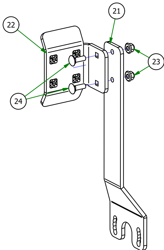
026-0019-01 Foot Pedal Assembly
