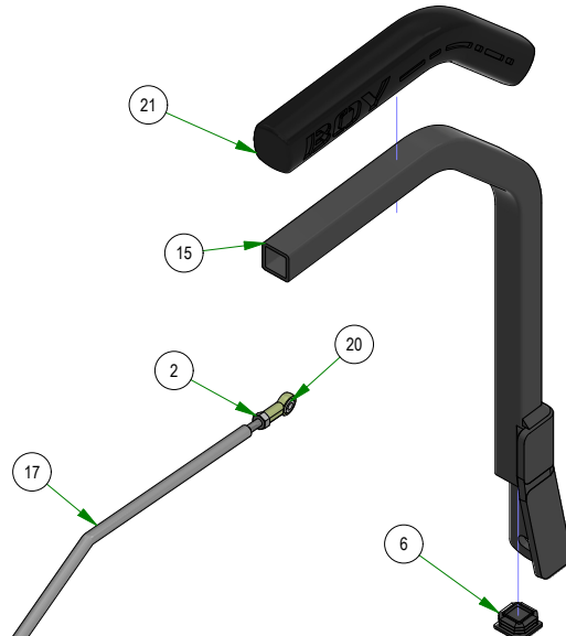
031-9071-00 LEFT DRIVE ARM
